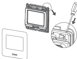
Рисунок 18. Схема сборки терморегулятора
